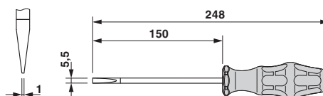
Desenho de medidas
