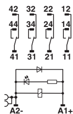
Diagrama de circuitos
