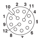
Imagem com polos soquete M12, 12 polos, vista lado do soquete
