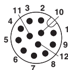
Imagem com pólos plugue M12, 12 pólos, vista lado do pino
