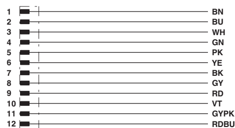
Esquema de ligação do conector M12
