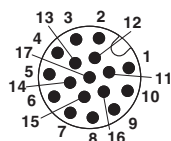
Imagem com pólos plugue M12, 17 pólos, vista lado do pino
