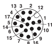
Imagem com pólos plugue M12, 17 pólos, vista lado do pino
