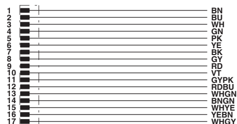
Esquema de ligação do conector M12
