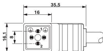
Conector para válvula, formato C
