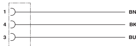
Esquema de ligação do soquete M12
