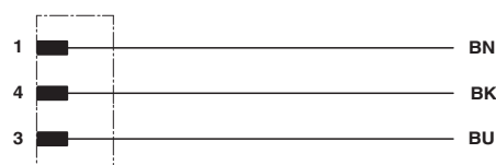
Esquema de ligação do conector M12
