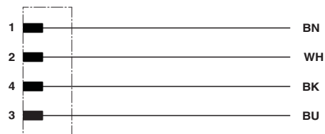
Alocação de conexão do plugue M8
