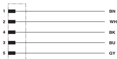
Diagrama de circuitos
