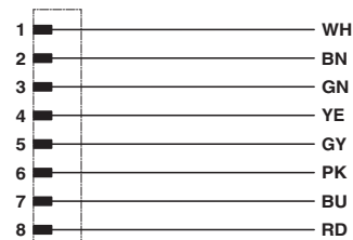
Diagrama de circuitos
