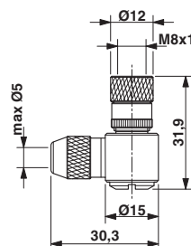
Desenho de medidas
