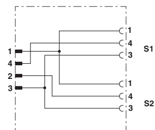
Alocação de conexão do distribuidor Y M8
