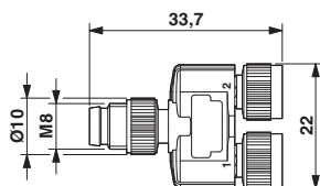
Desenho de medidas
