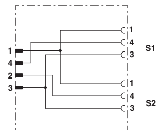
Alocação de conexão do distribuidor Y M12/M8
