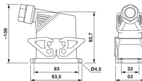
Imagem dimensional
