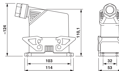
Imagem dimensional
