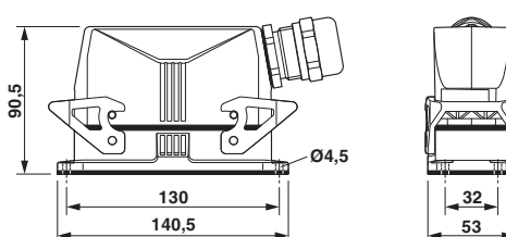
Imagem dimensional
