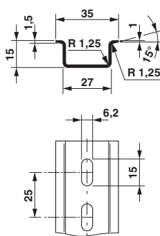
Desenho de medidas
