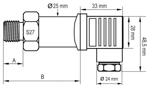
Fig. 5 – Dimensões do transmissor
