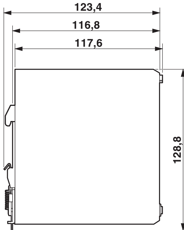
Desenho de medidas
